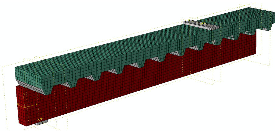
Fig. 4. Mesh
